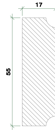
Detalje: Fenderliste
